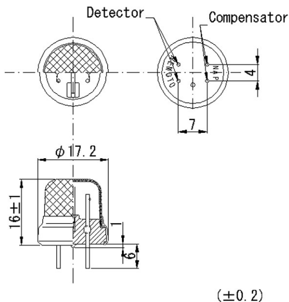
図 NCP-300S の外観、寸法
