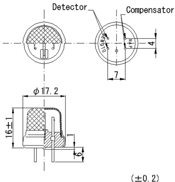
図 NCP-180S-N の外観、寸法
