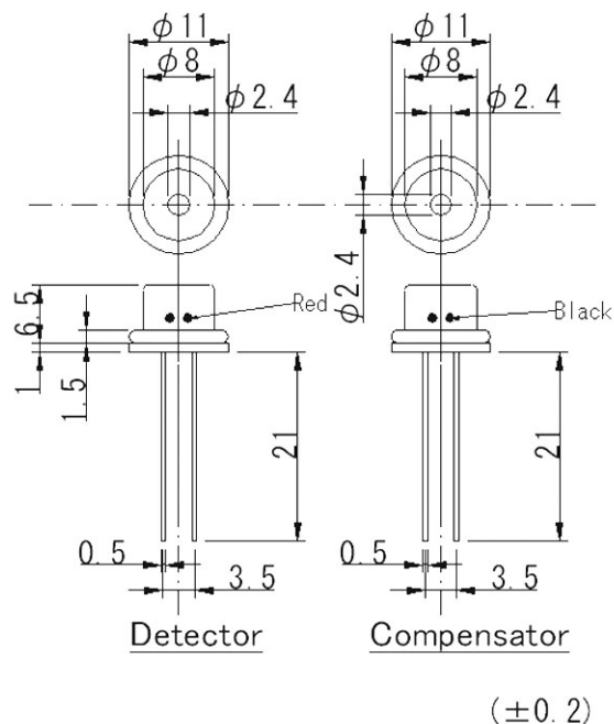
図 NCP-180 の外観、寸法
