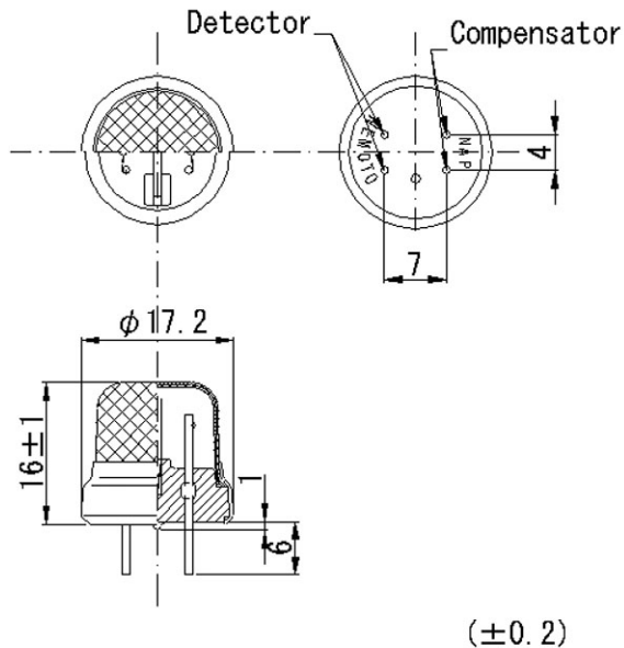
図 NCP-180S-H の外観、寸法
